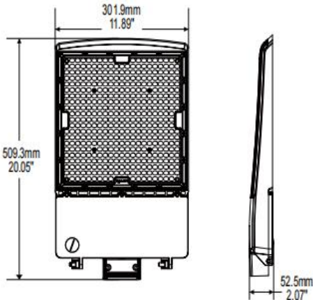
240W&300W
